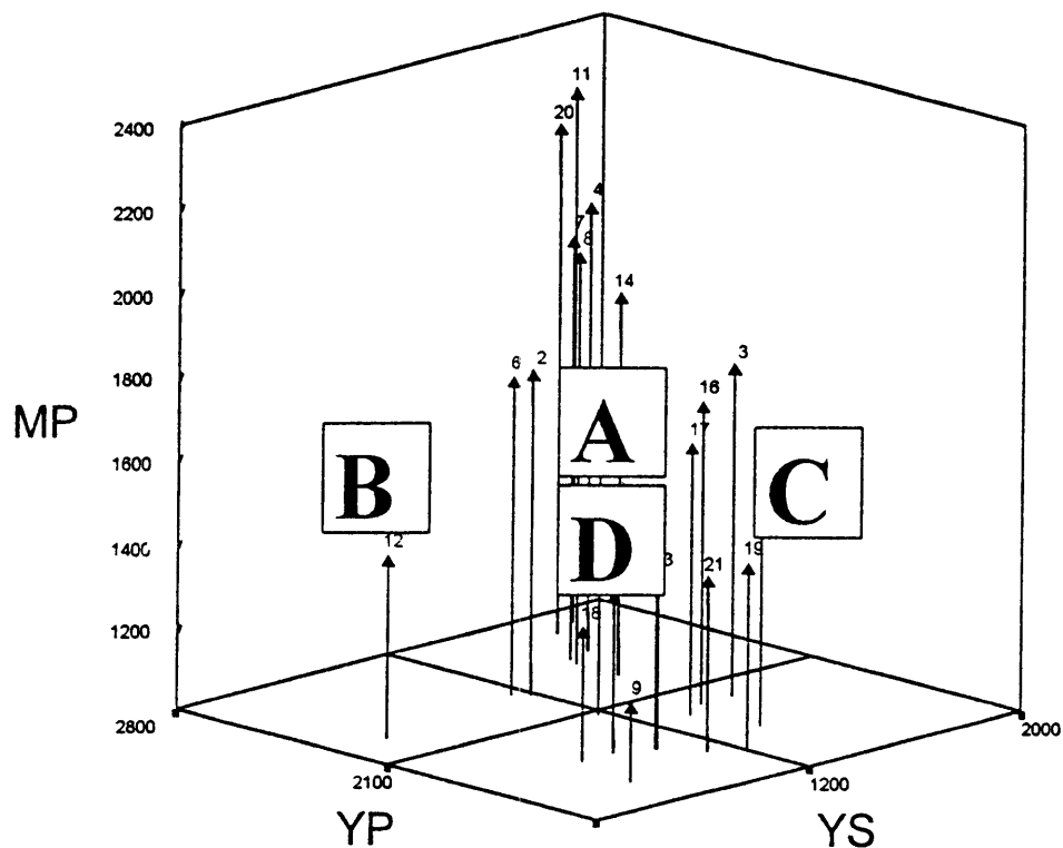
شکل ۳- نمودار سه بعدی تعیین ارقام به خشکی بر اساس عملکرد آبی (Yp)، عملکرد دیم (Ys) و شاخص MP
