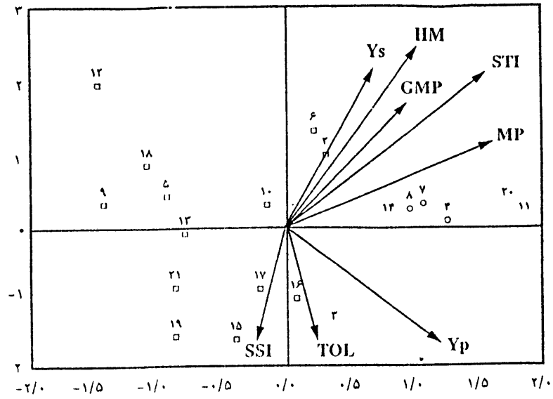
شکل ۵- نمایش بای پلات ۲۱ لاین نخود ایرانی در ۸ شاخص مقاومت به خشکی براساس اولین و دومین مؤلفه اصلی
